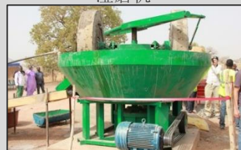
湿磨机
